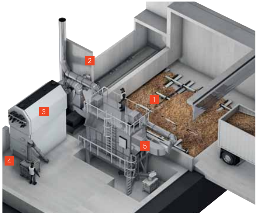
Anwendungsbeispiel Vitoflex 300-FSB
